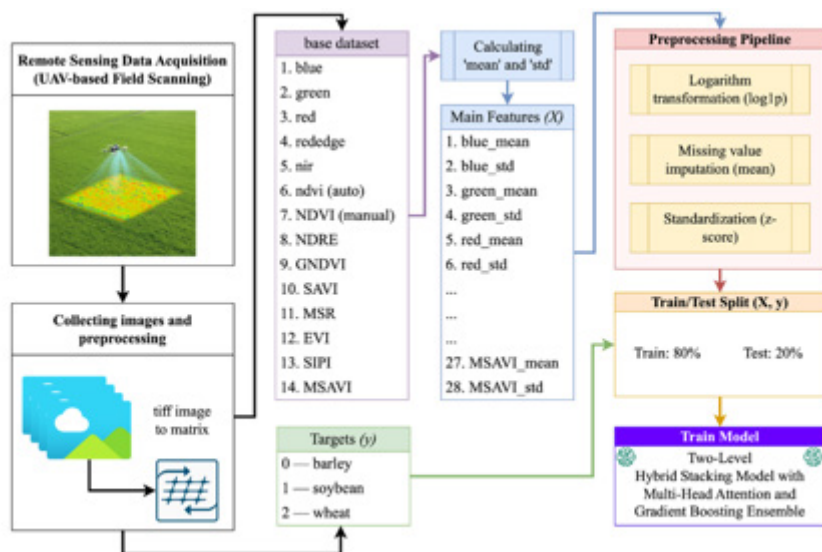
Сур. 1. UAV мультиспектралды деректер негізінде дақылдарды жіктеуге арналған деректерді өңдеу және гибридісті стекинг-модельді бар талдау пайплайны
