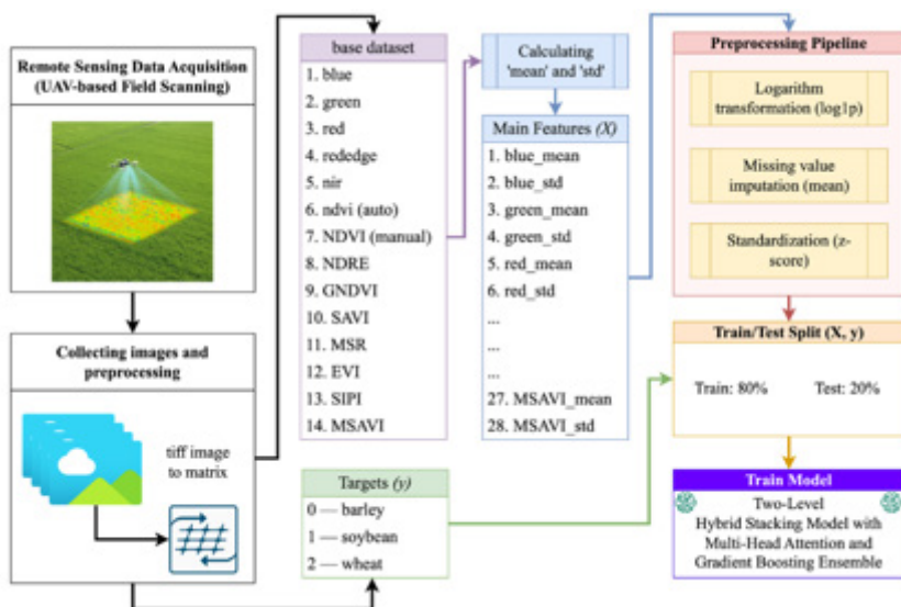
Сур. 1. UAV мультиспектралды деректер негізінде дақылдарды жіктеуге арналған деректерді өңдеу және гибридісті стекинг-моделі бар талдау пайплайны
