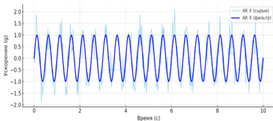
Рис. 1. Вибрации по оси X: до и после фильтрации
